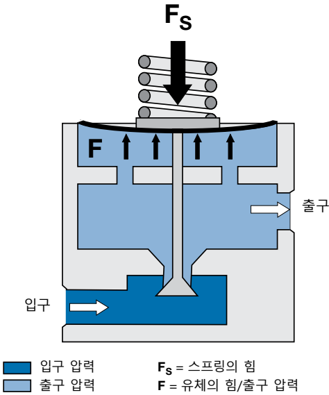
감압 레귤레이터
